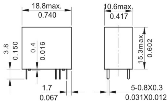
外形尺寸图 Dimensions
